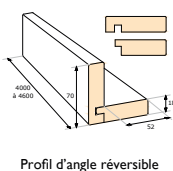
Profil d'angle réversible
